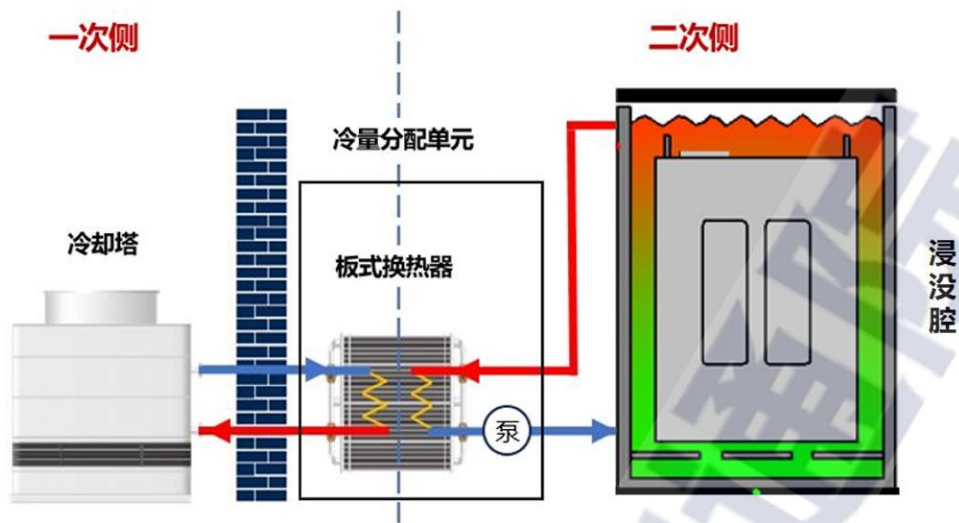
图 浸没式液冷系统原理图
