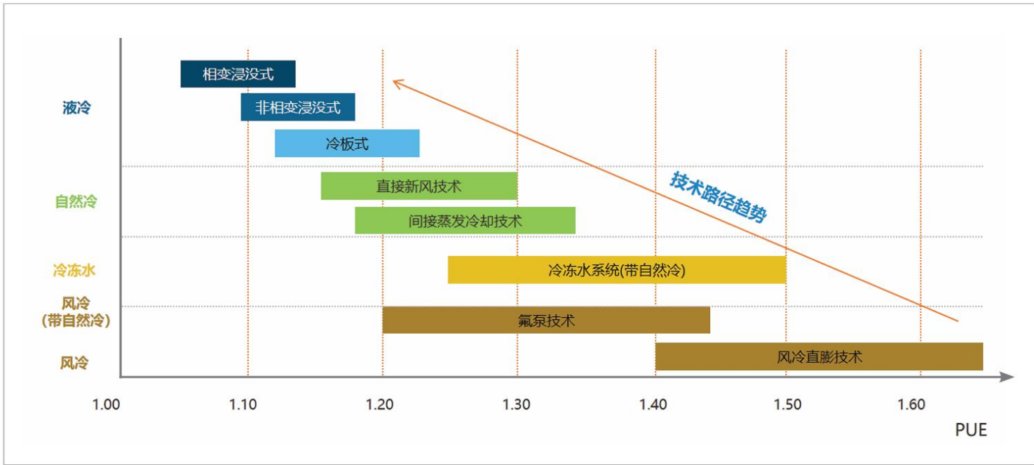
图 数据中心制冷技术对应PUE范围
