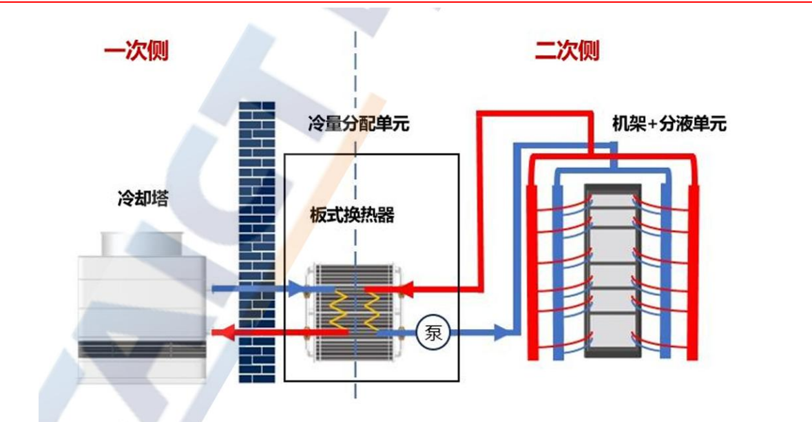
图 冷板式液冷系统原理图
