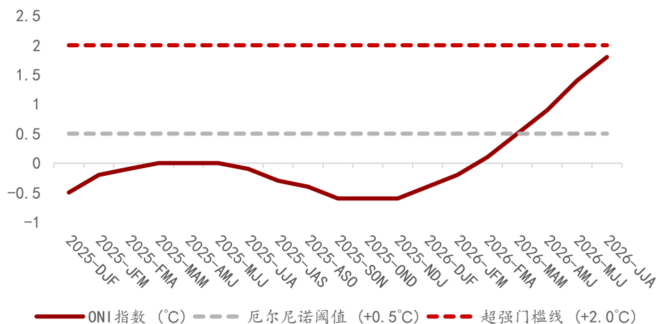
图表7: 2025-2026年厄尔尼诺指数 (ONI) 月度演变图
