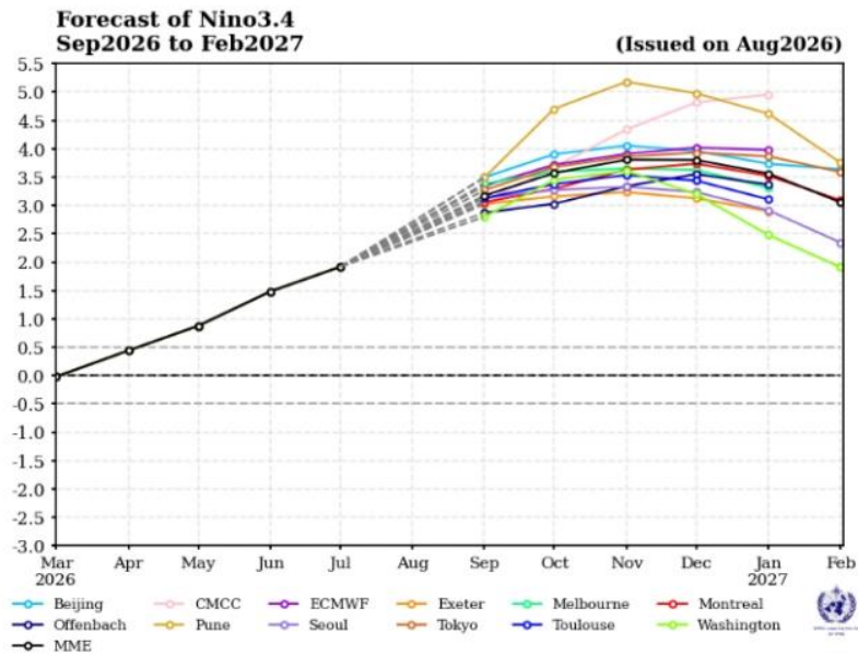
图表10：2026年9月至2027年2月Niño3.4区多模型预测图
