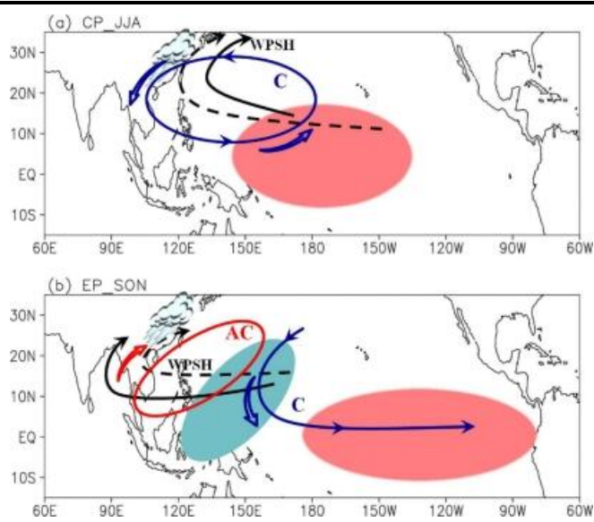
图表14: El Nino在发展期影响我国降水的物理过程
