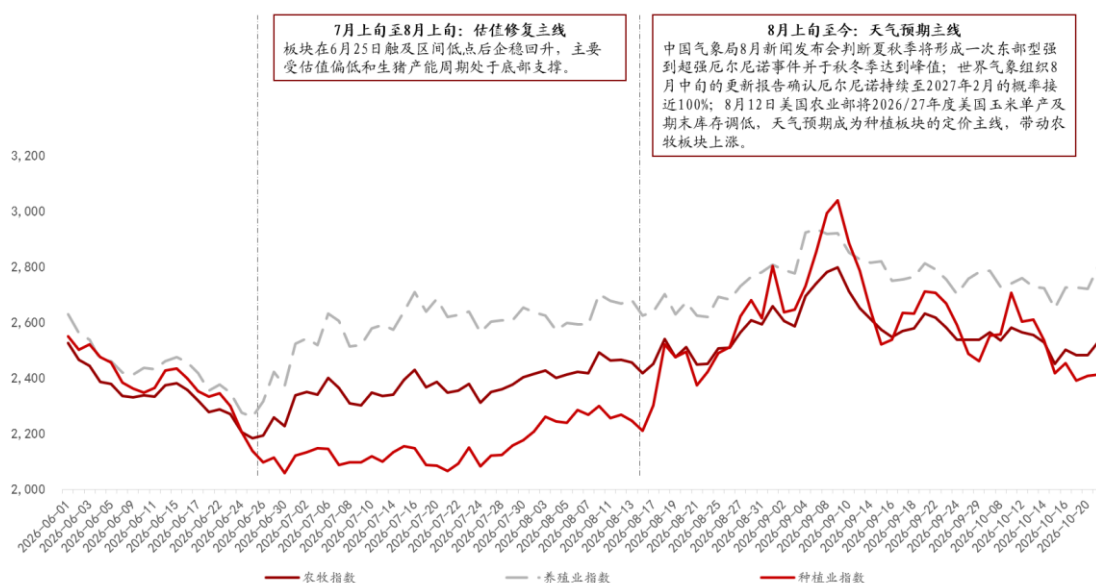
图表2：本轮农牧行情可大致分为估值修复及天气预期两大阶段
