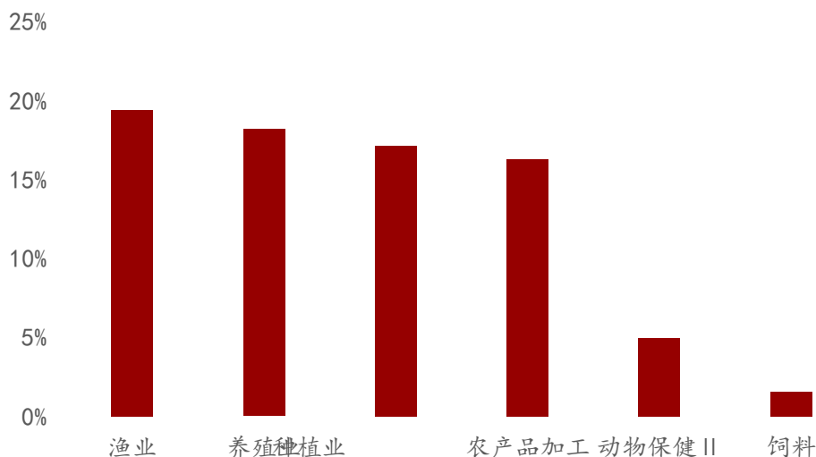
图表3：农牧子板块分化明显，涨幅呈清晰梯度
