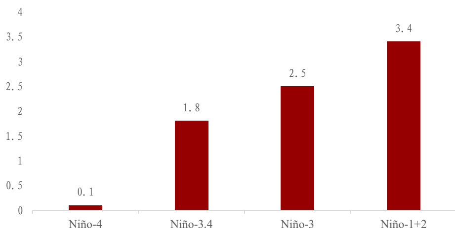
图表8: 2026年8月四大Niño监测区海温距平对比 (°C)
