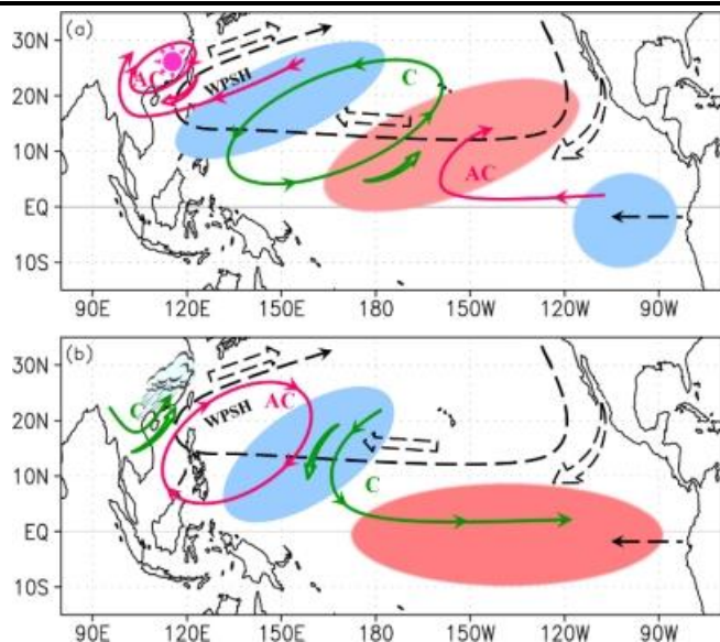
图表13: El Nino在衰退期影响我国降水的物理过程
