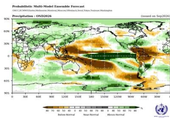
图表12：2026年10-11-12月全球降水概率预测图
