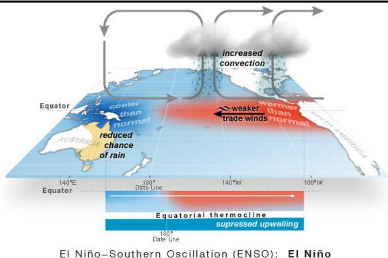
图表6: ENSO大气环节--厄尔尼诺年份沃克环流截面
