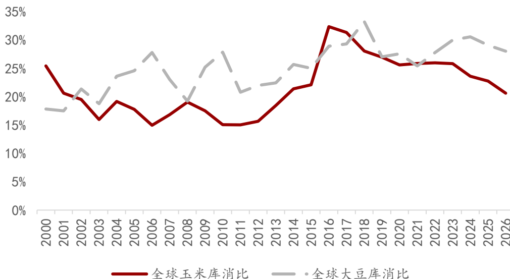
图表20：玉米库消比处于历史低位，而大豆库消比则相对健康
