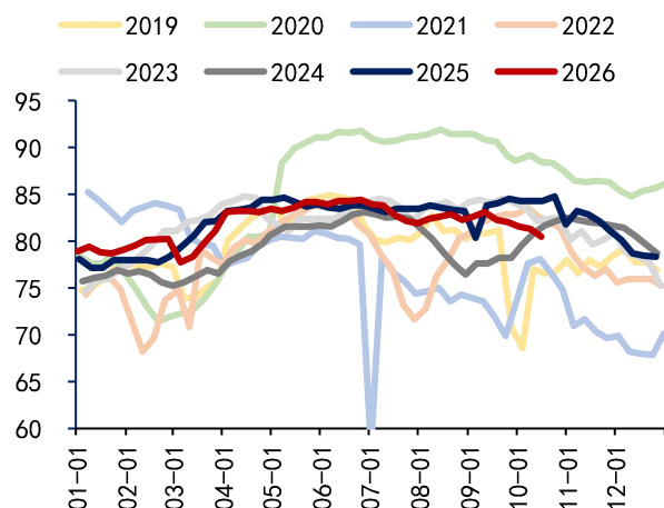
图表 1 全国高炉开工率（247 家）
