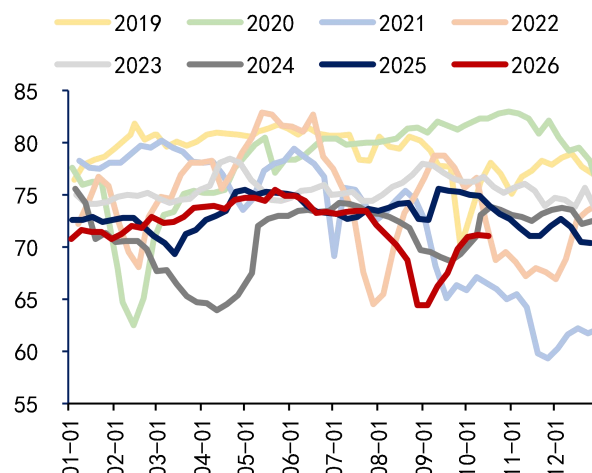
图表 2 中国:焦炉生产率:国内独立焦化厂(230 家)
