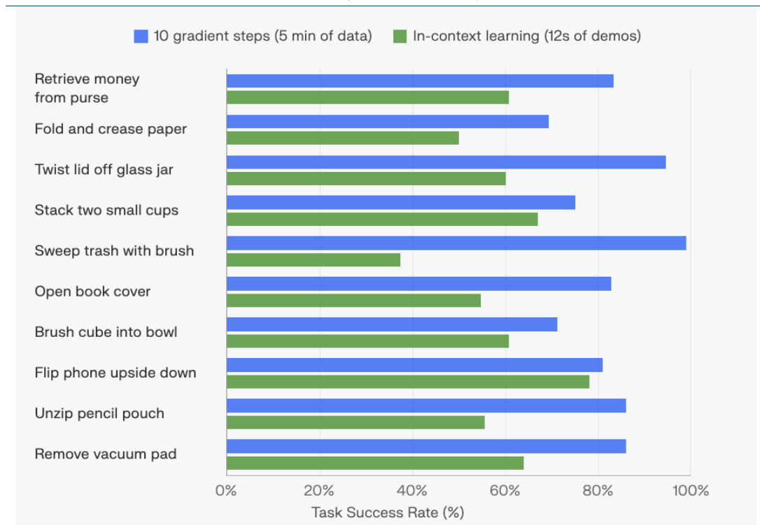
图表2: GEN-1.5 一次性上下文学习与少样本后训练成功率对比
