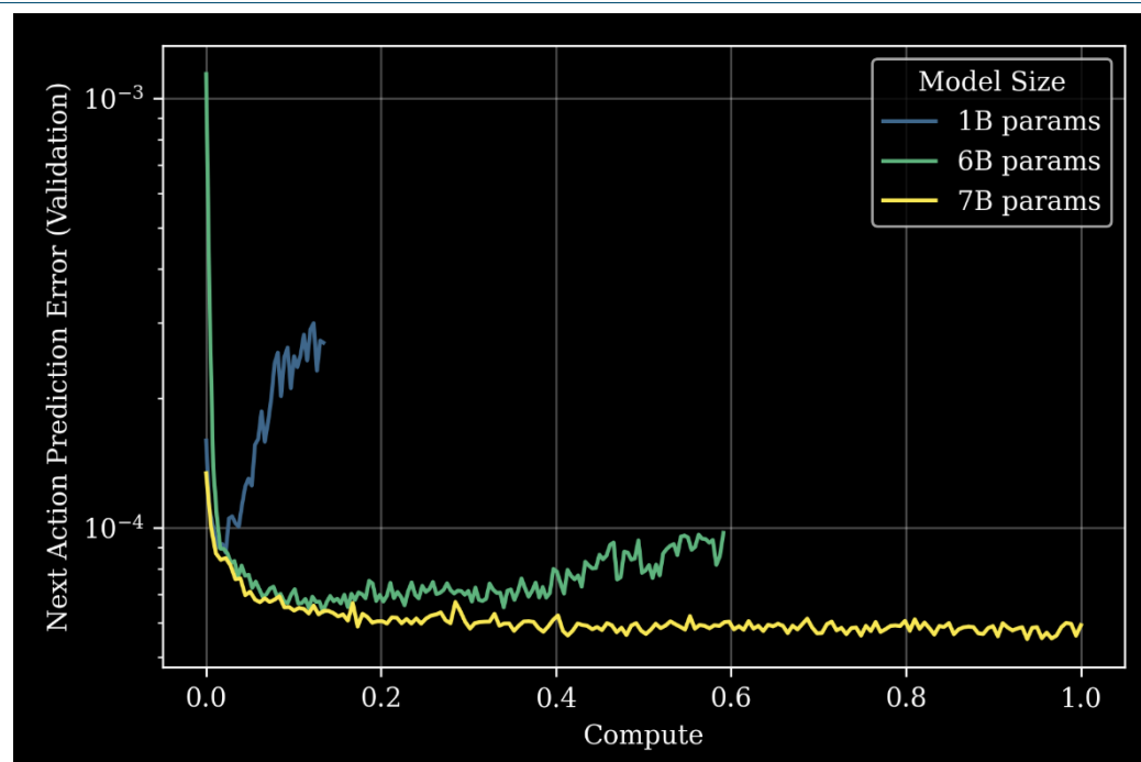
图表3: GEN-0 不同参数量模型的预训练表现对比
