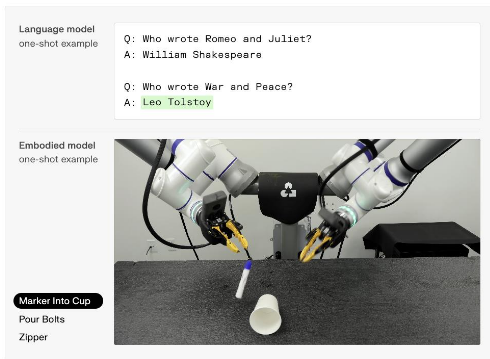
图表1：语言模型与具身模型上下文学习方式对比
