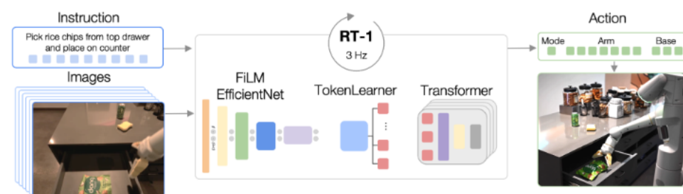
图表14: Google RT-1 架构
