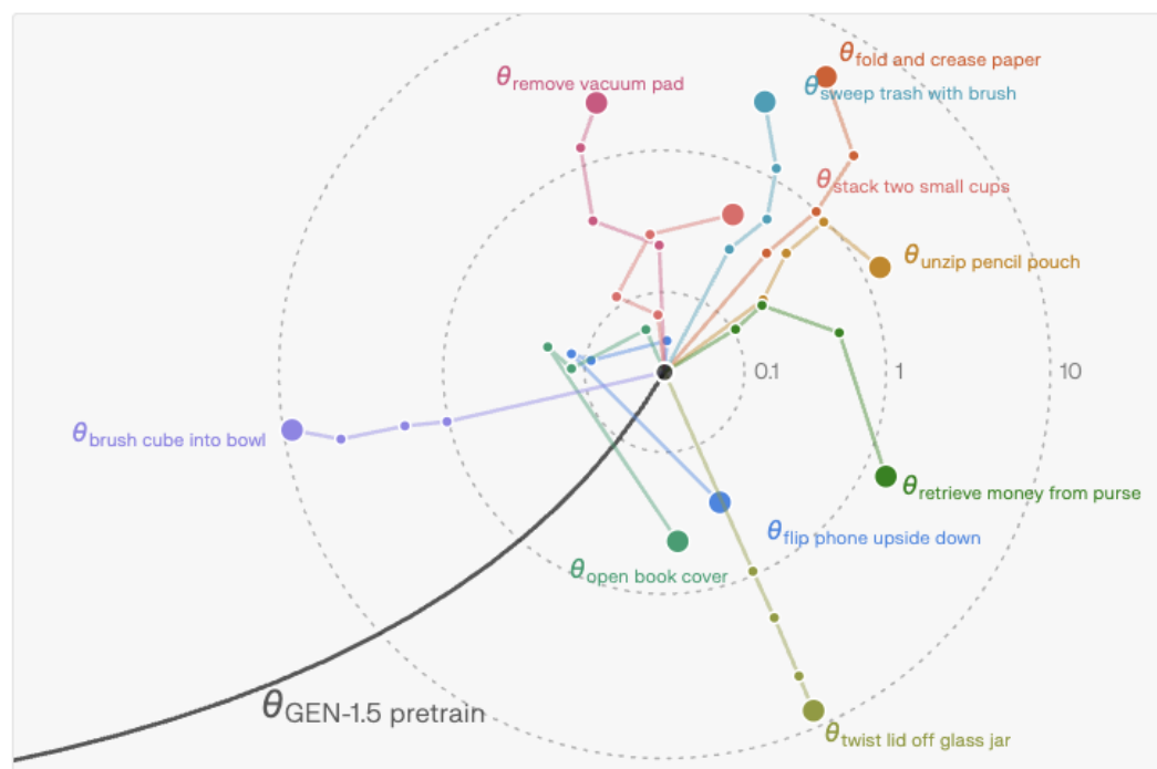
图表7: GEN-1.5 仅需 1-10 个梯度步即可适配新任务
