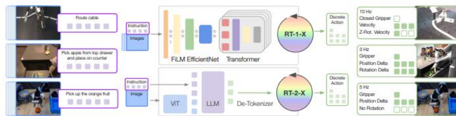
图表16: Google RT-1-X 与 RT-2-X 架构图
