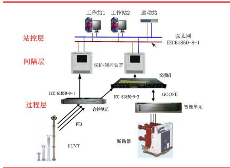
图 10:变电站智能化结构图
